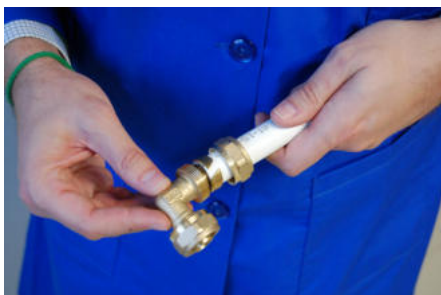
3. Acoplar tubo y accesorio según se muestra 3. Acoplamento de tubos e acessório, como mostrado
