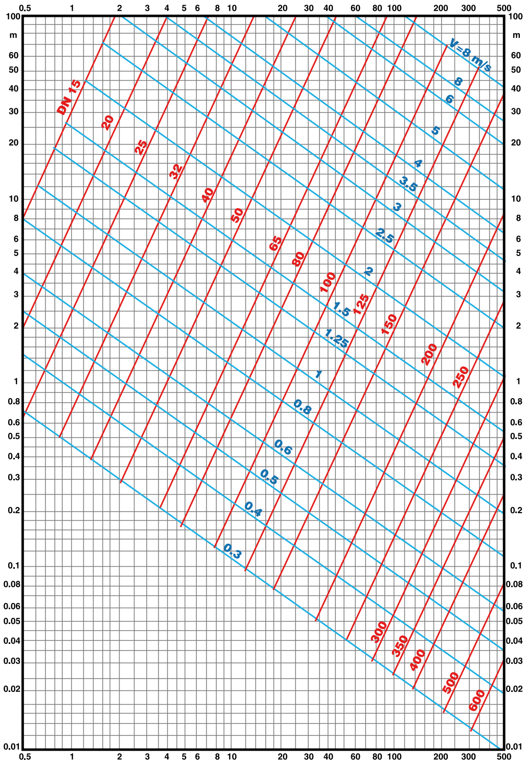
Pérdida de carga Hv por cada 100 m. de tubería.
