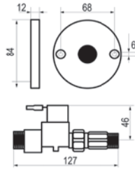
Sistema completo (detector+electroválvula)
