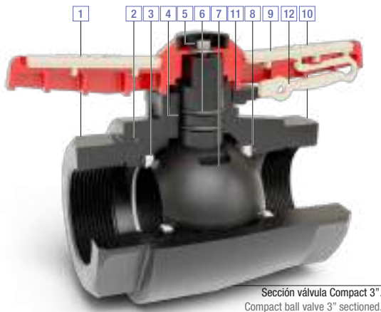
Sección válvula Compact. Compact ball valve sectioned.
