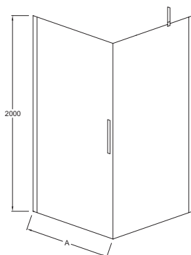
Dibujo correspondiente a mamparas de 70, 80 y 90 cm.
