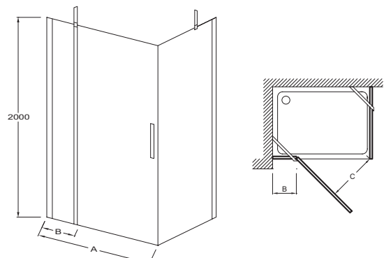
Dibujo correspondiente a mamparas de 100, 110 y 120 cm.
