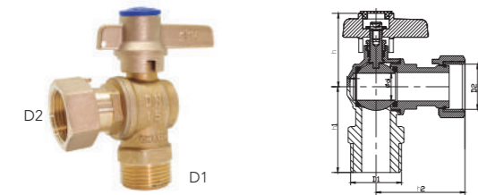
VÁLVULA SALIDA ESCUADRA ROSCA BSP M-H ISO 228/1. Palanca. Tuerca loca. Con retención interior
